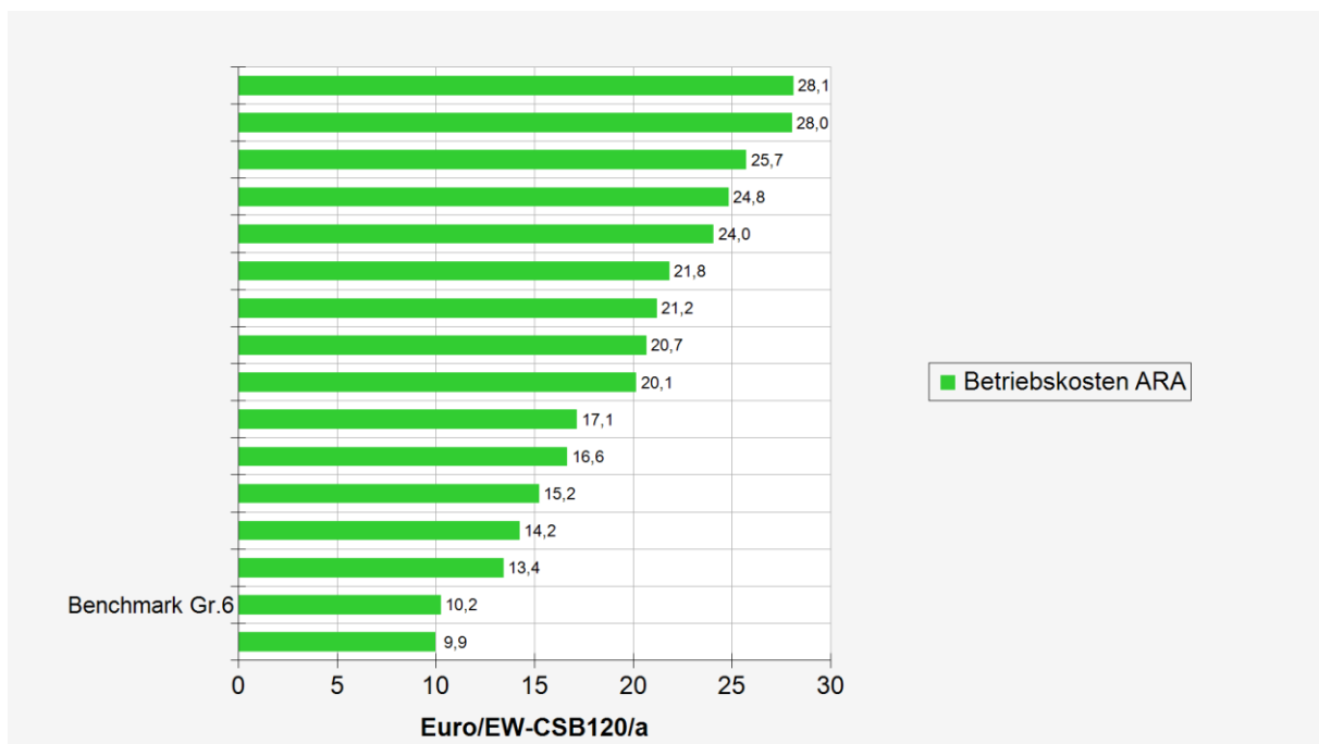
Abbildung 28: Betriebskosten der Kläranlagen der Gruppe 6
