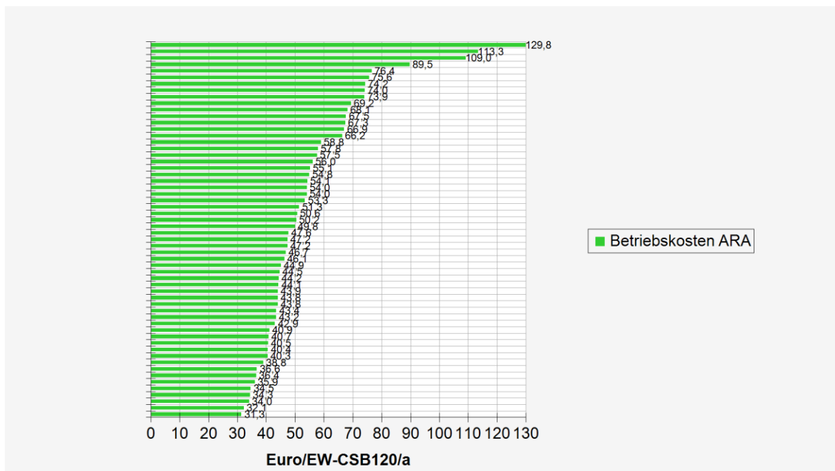
Abbildung 8: Betriebskosten der Kläranlagen der Gruppe 1
