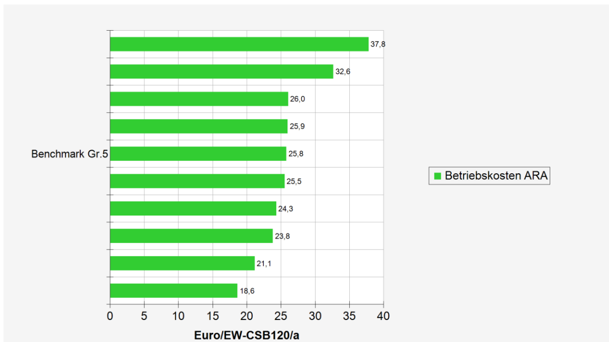
Abbildung 24: Betriebskosten der Kläranlagen der Gruppe 5
