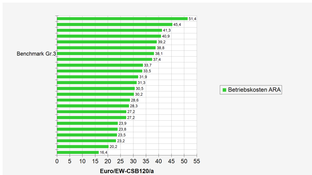
Abbildung 16: Betriebskosten der Kläranlagen der Gruppe 3
