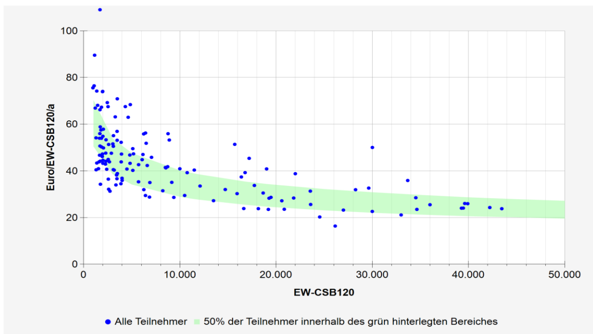
Abbildung 6: BM-Kostenkurve der spez. Betriebskosten
