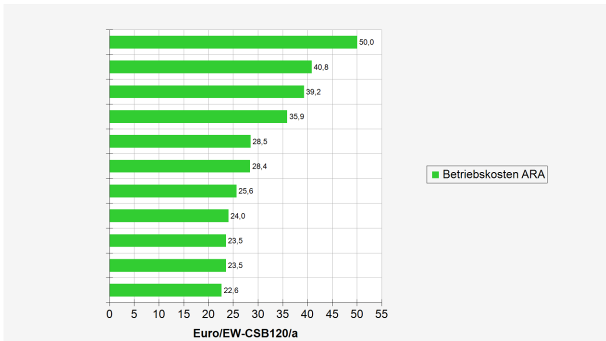
Abbildung 20: Betriebskosten der Kläranlagen der Gruppe 4
