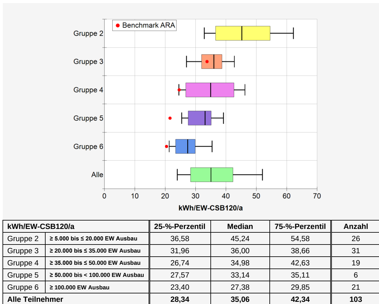
Abbildung 3: Vergleich des elektrischen Energieverbrauchs
