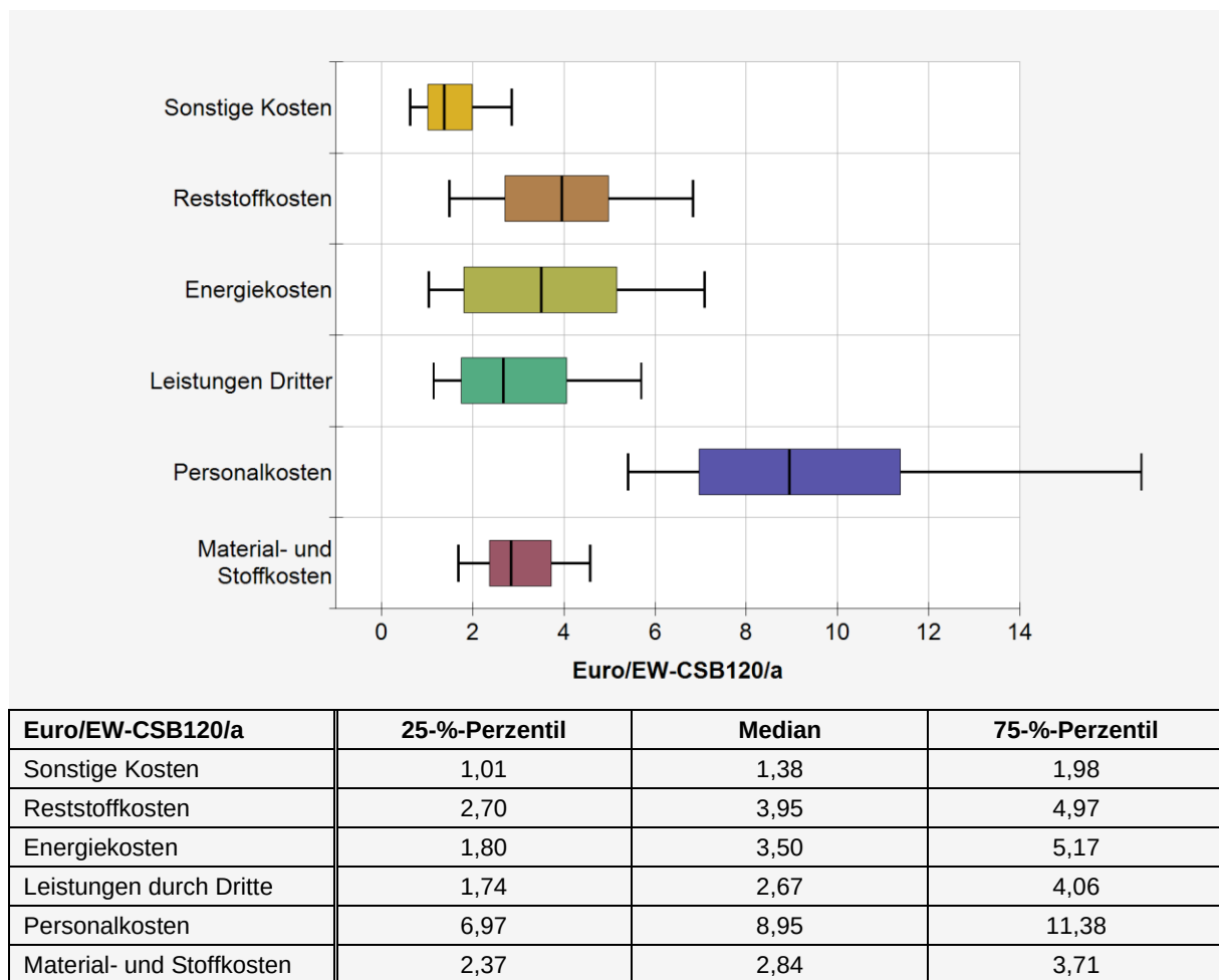
Abbildung 1: Kostenverteilung nach Hauptkostenarten der Kläranlage
