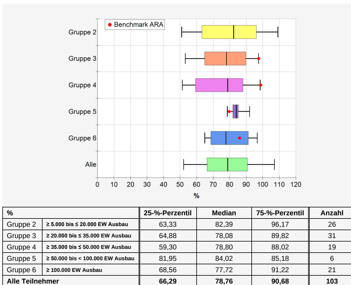
Abbildung 4: Vergleich der Auslastung
